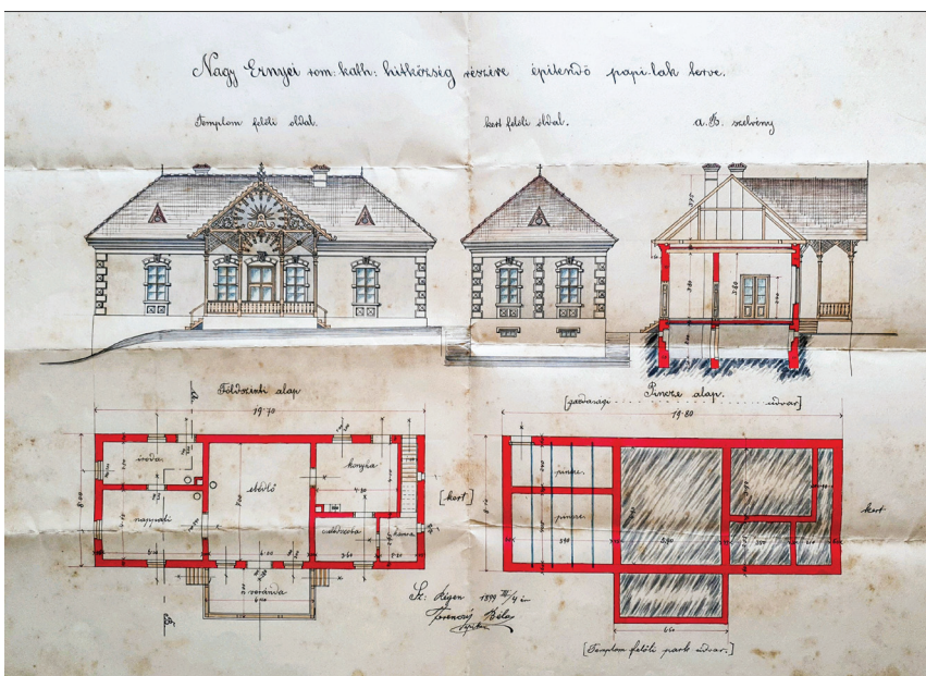
A nagyernyei papi lak építési tervrajza (1899)
