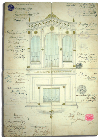
Kolonics István szabadkai orgonaépítő szignált orgonarajza (1888)
