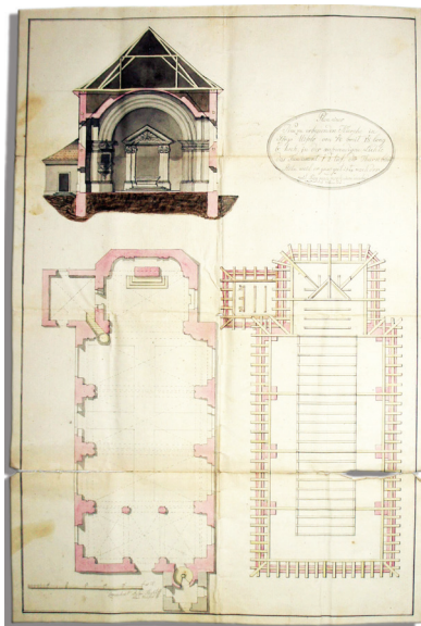
A gyergyóújfalvi templom tervrajza (1824)
